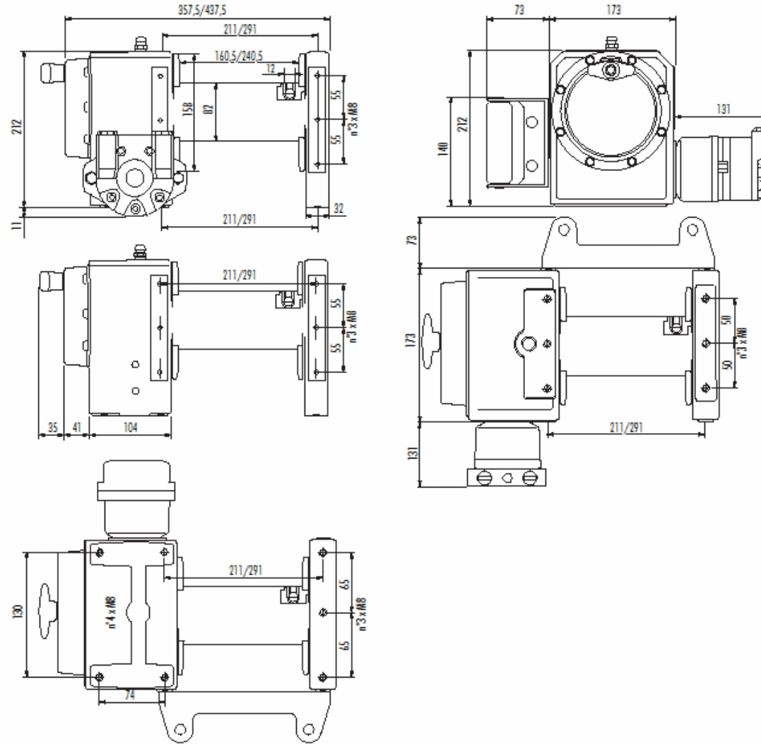
Abmessungen mit Kompakthydraulikmotor
